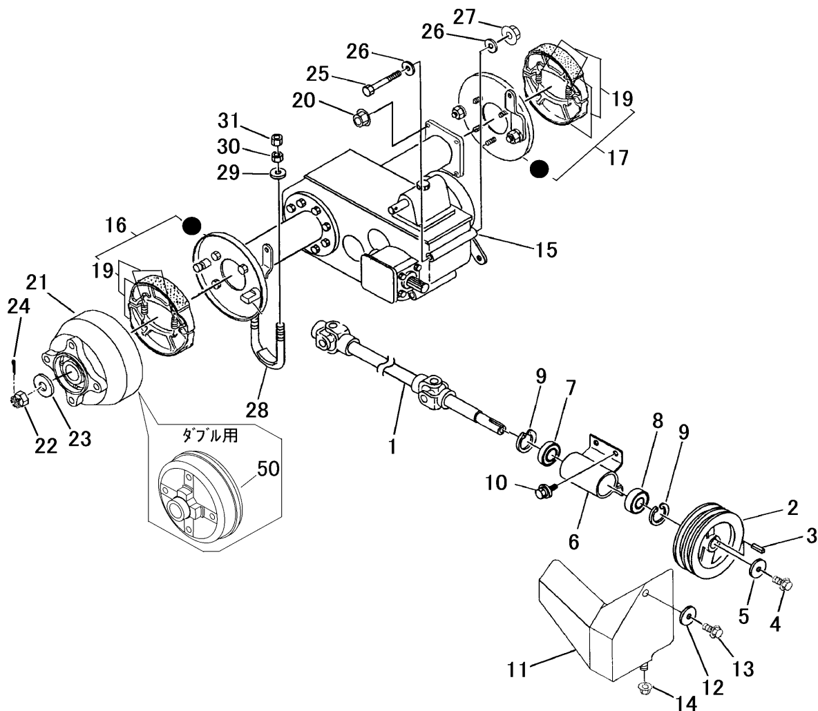
FIG 6 プロペラシャフト & ミッション PROPELLERSHAFT & TRANSMISSION
