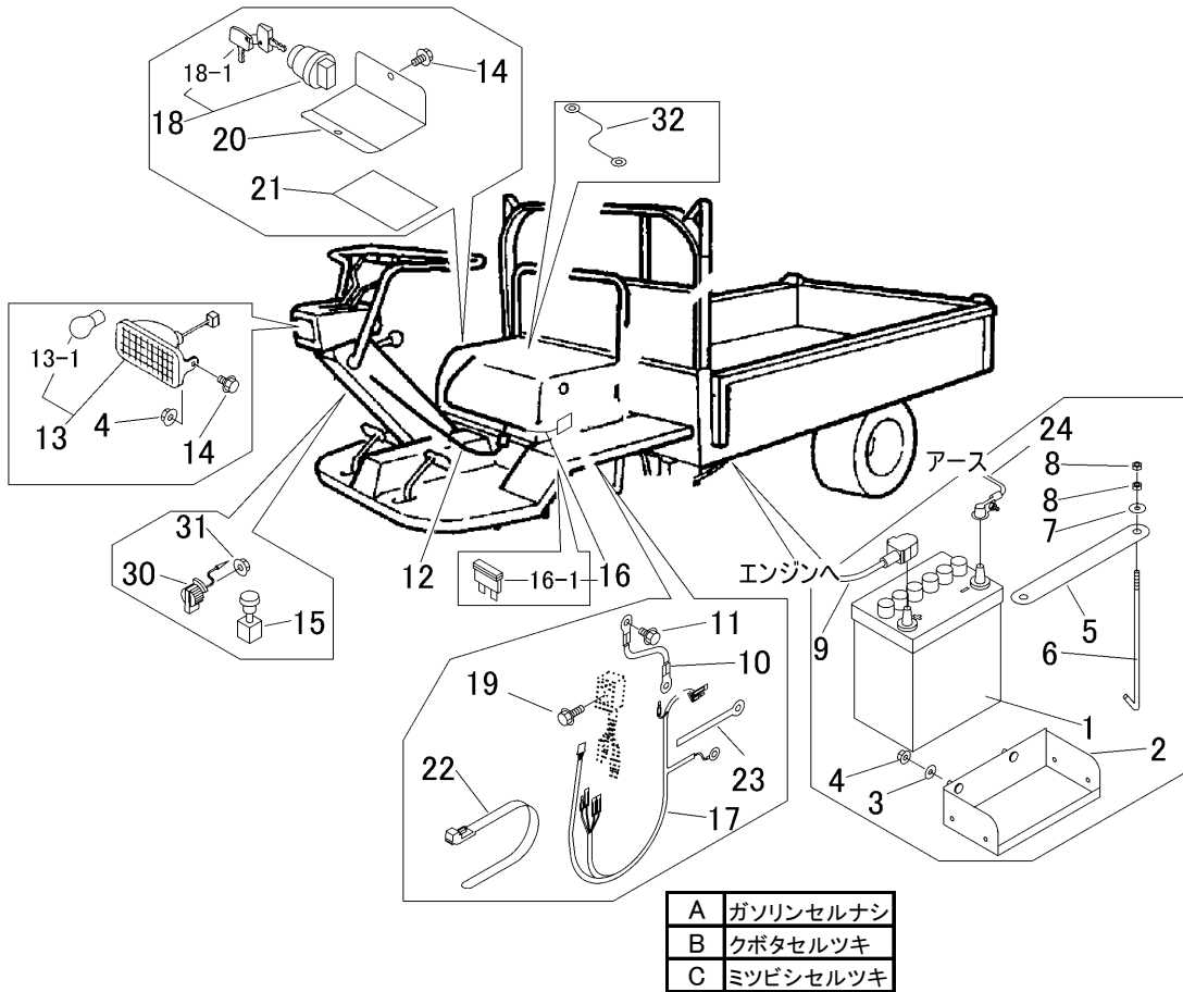
FIG 3 デンソー (ミツビシ・クボタ ガソリン) ELECTRIC EQUIPMENT
