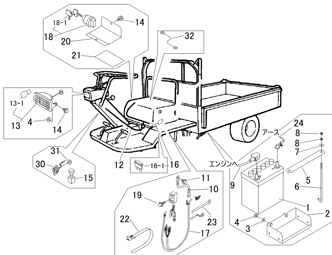
FIG 3 デンソー (ミツビシ・クボタ ガソリン) ELECTRIC EQUIPMENT
