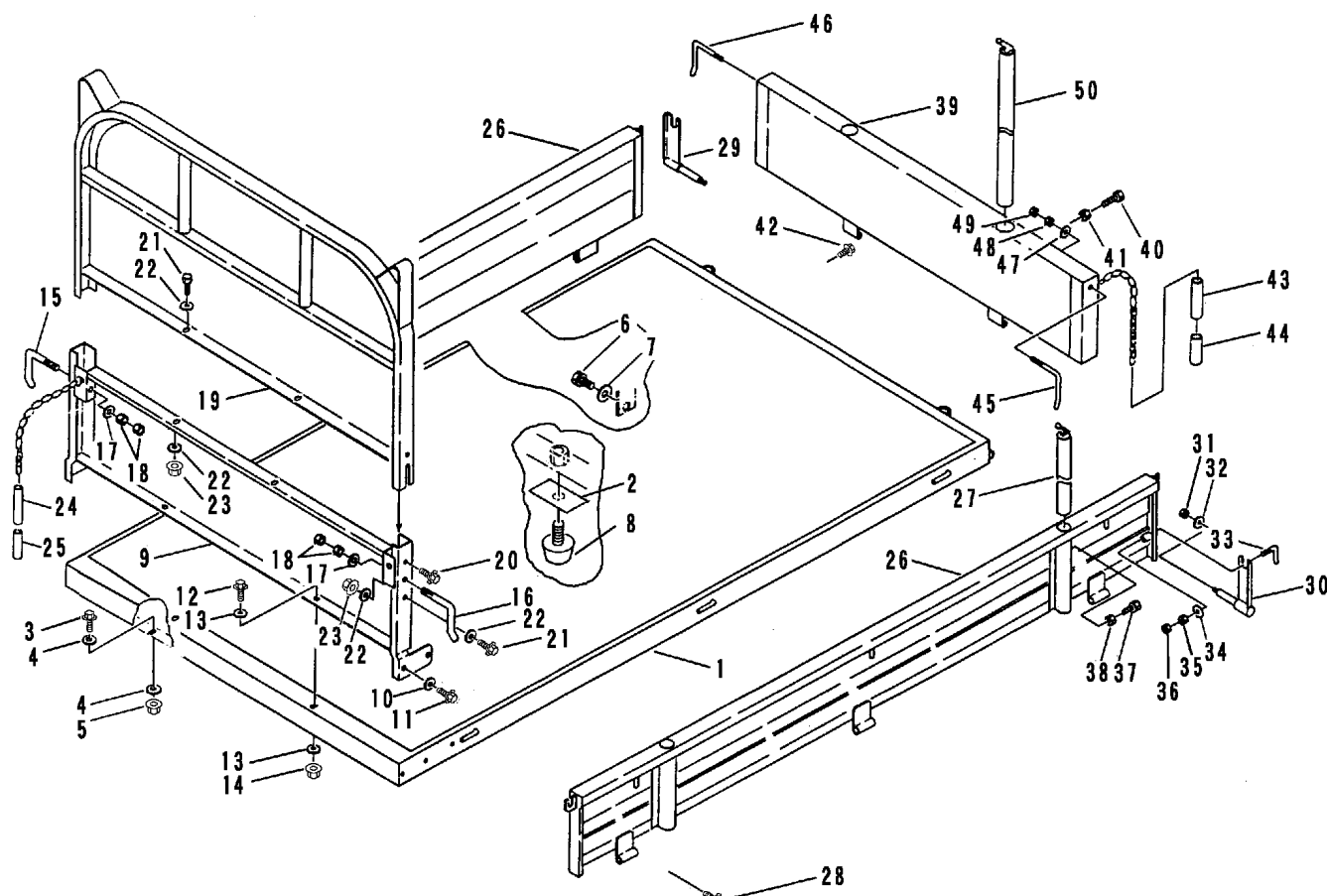
FIG 14 ニダイ & ドア (ショート荷台) WAGON & GATE
