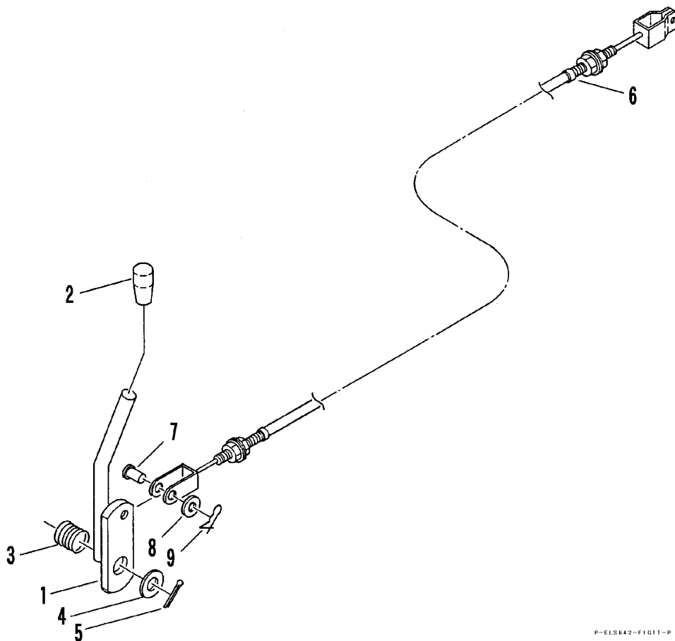
FIG 11 デフロック DIFFERENTIAL LOCK
