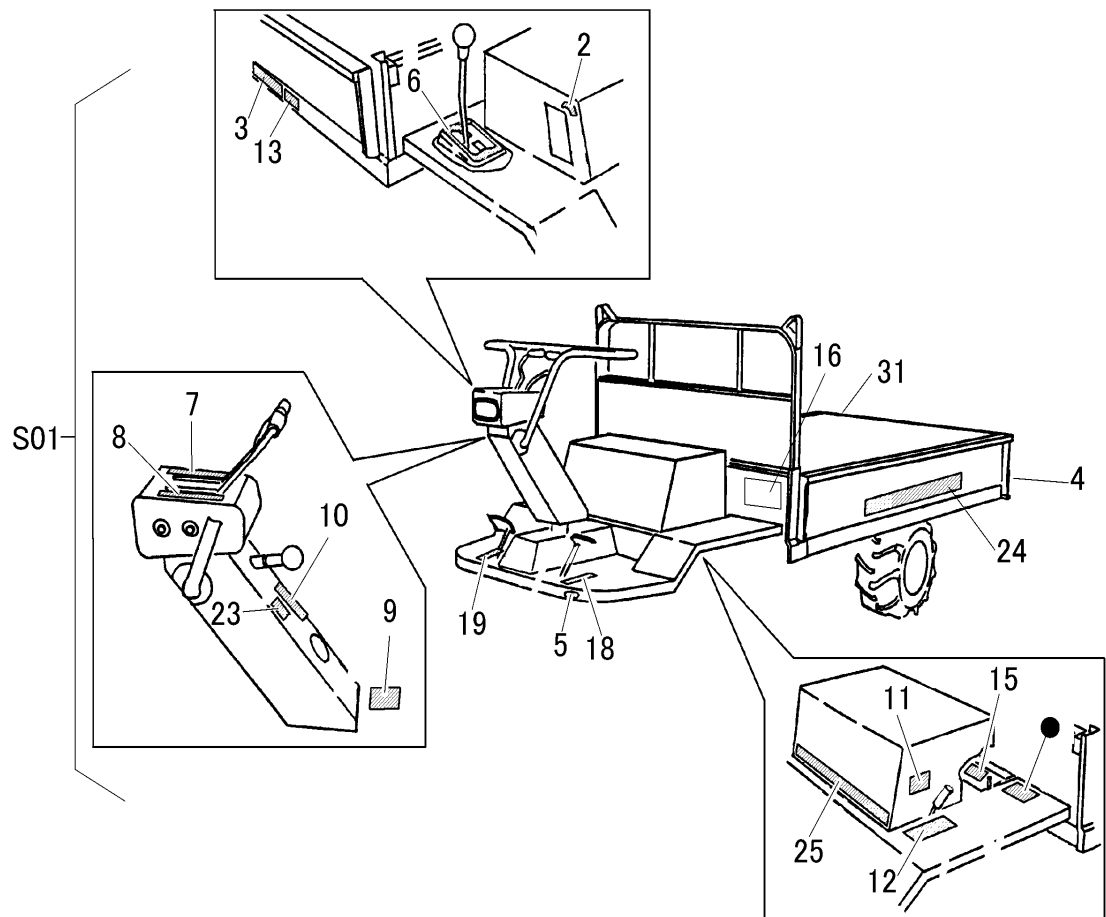
FIG 16 マーク (ミツビシ・クボタ ガソリン) MARK
