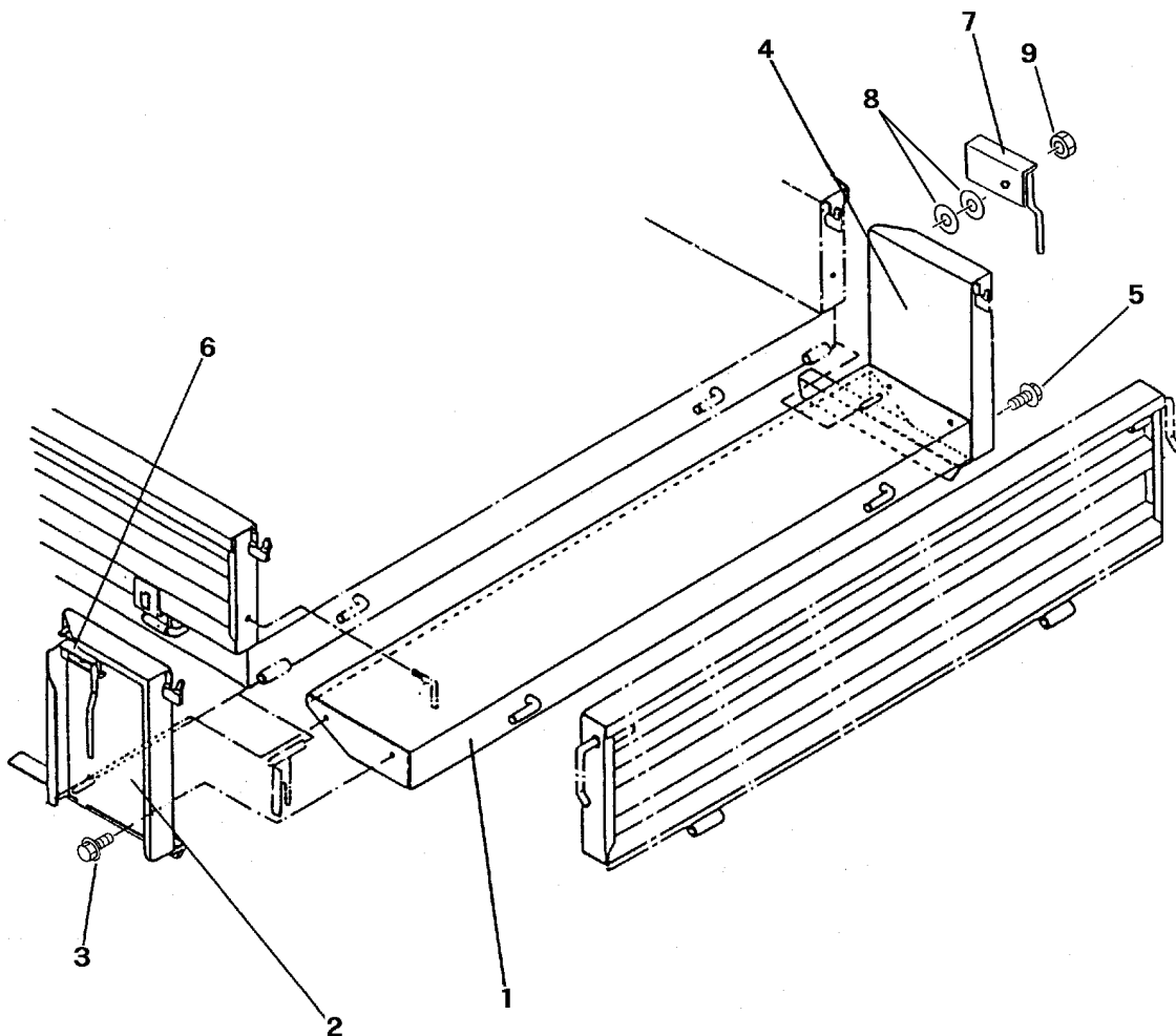
FIG 15 エンチョウニダイ OPTION
