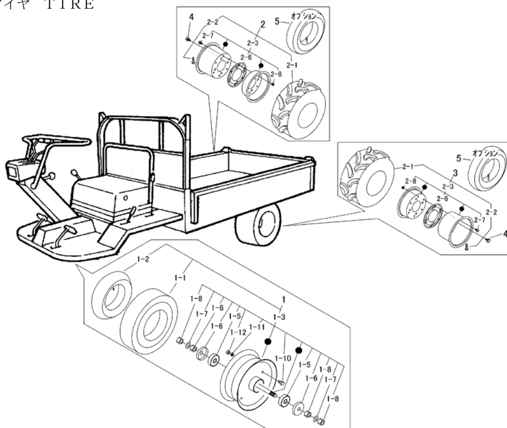
FIG 7 タイヤ TIRE
