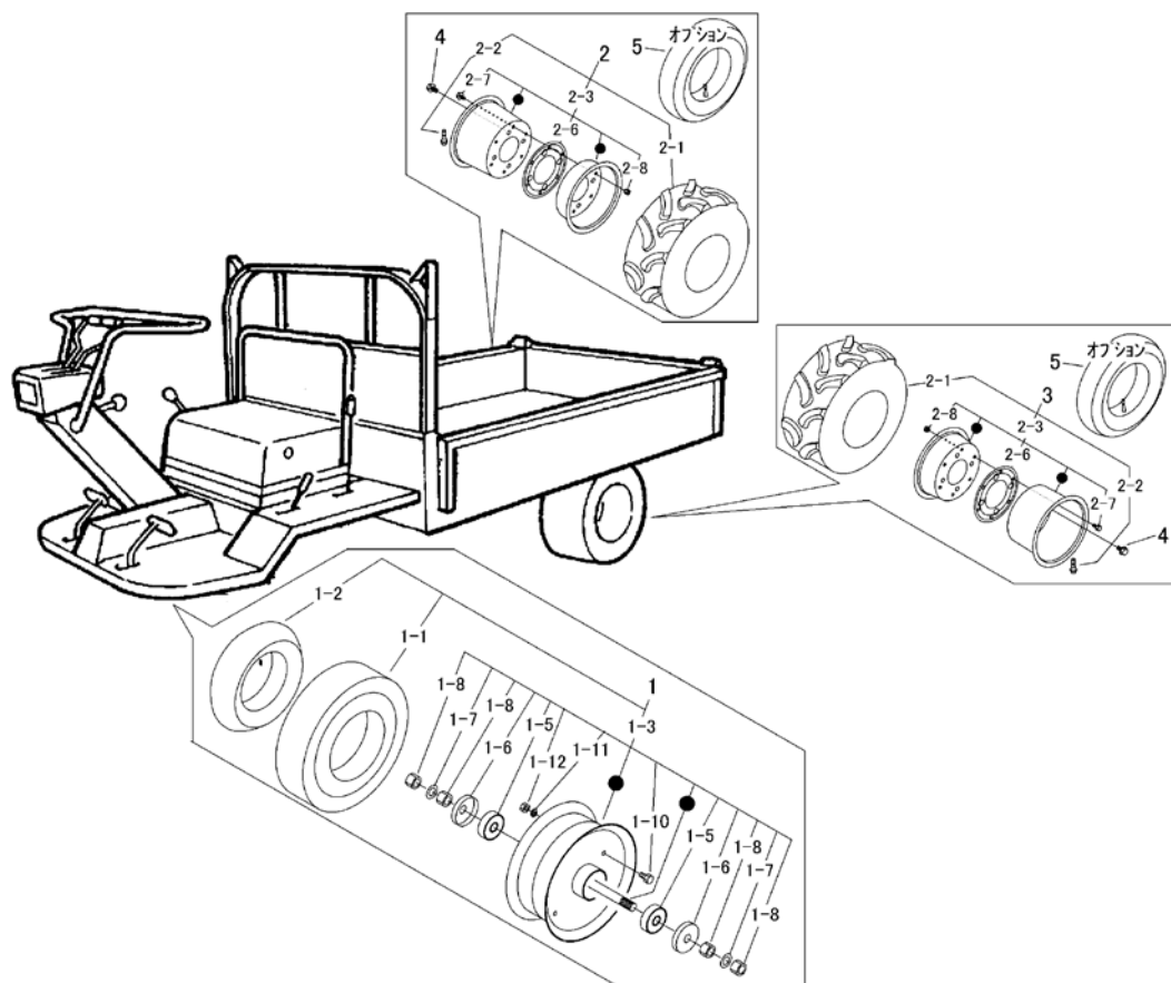
FIG 7 タイヤ TIRE
