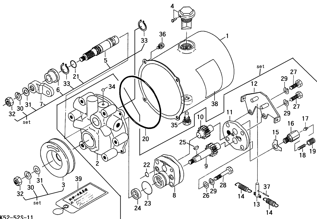
FIG 19 パッケージ H.Y.D PUMP ~NO.4161415
