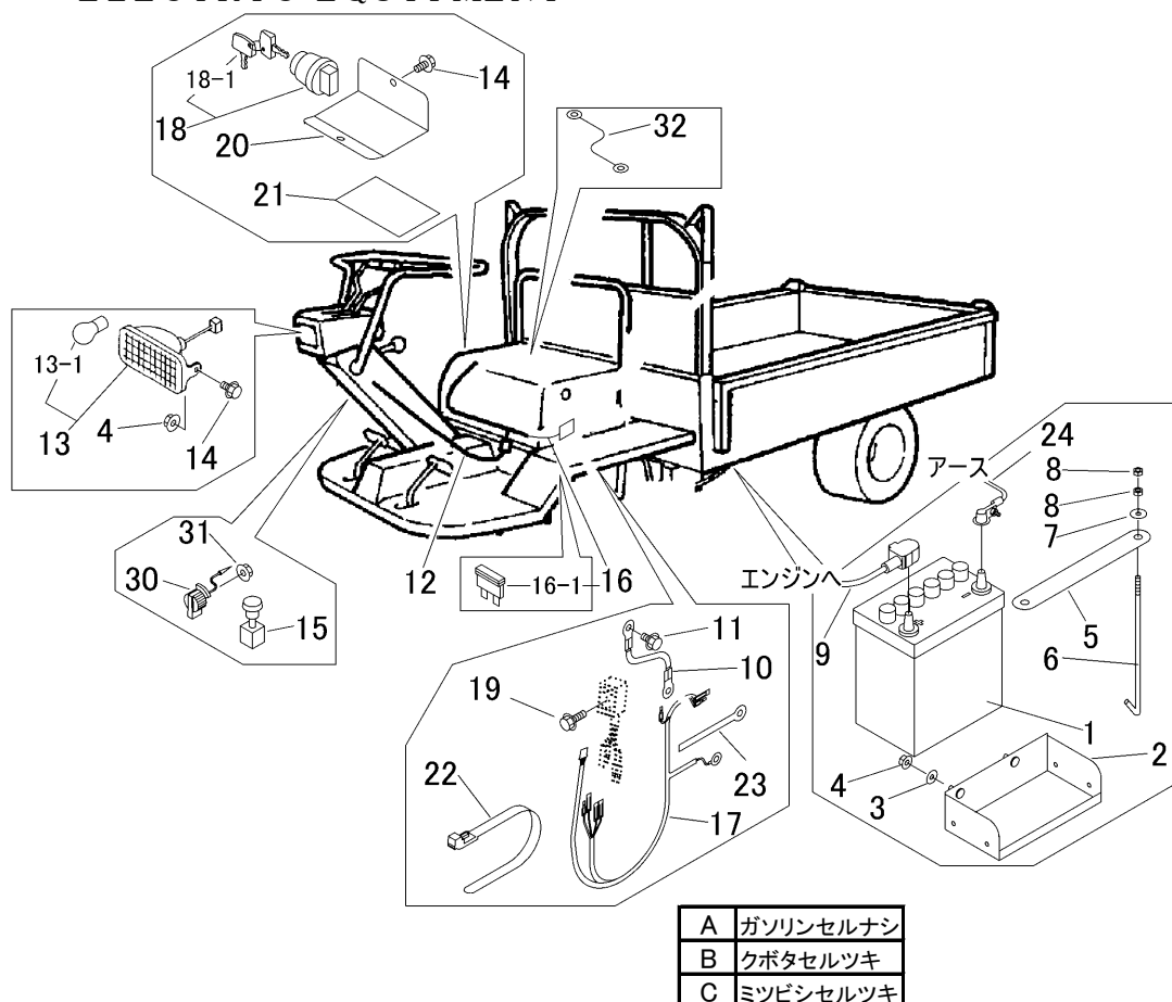
FIG 3 デンソー (ミツビシ・クボタ ガソリン) ELECTRIC EQUIPMENT
