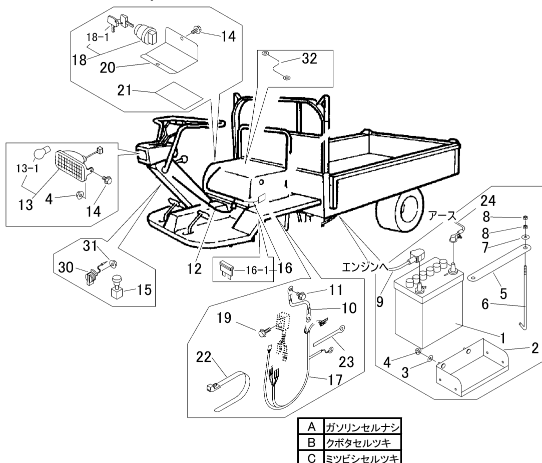
FIG 3 デンソウ (ミツビシ・クボタ ガソリン) ELECTRIC EQUIPMENT
