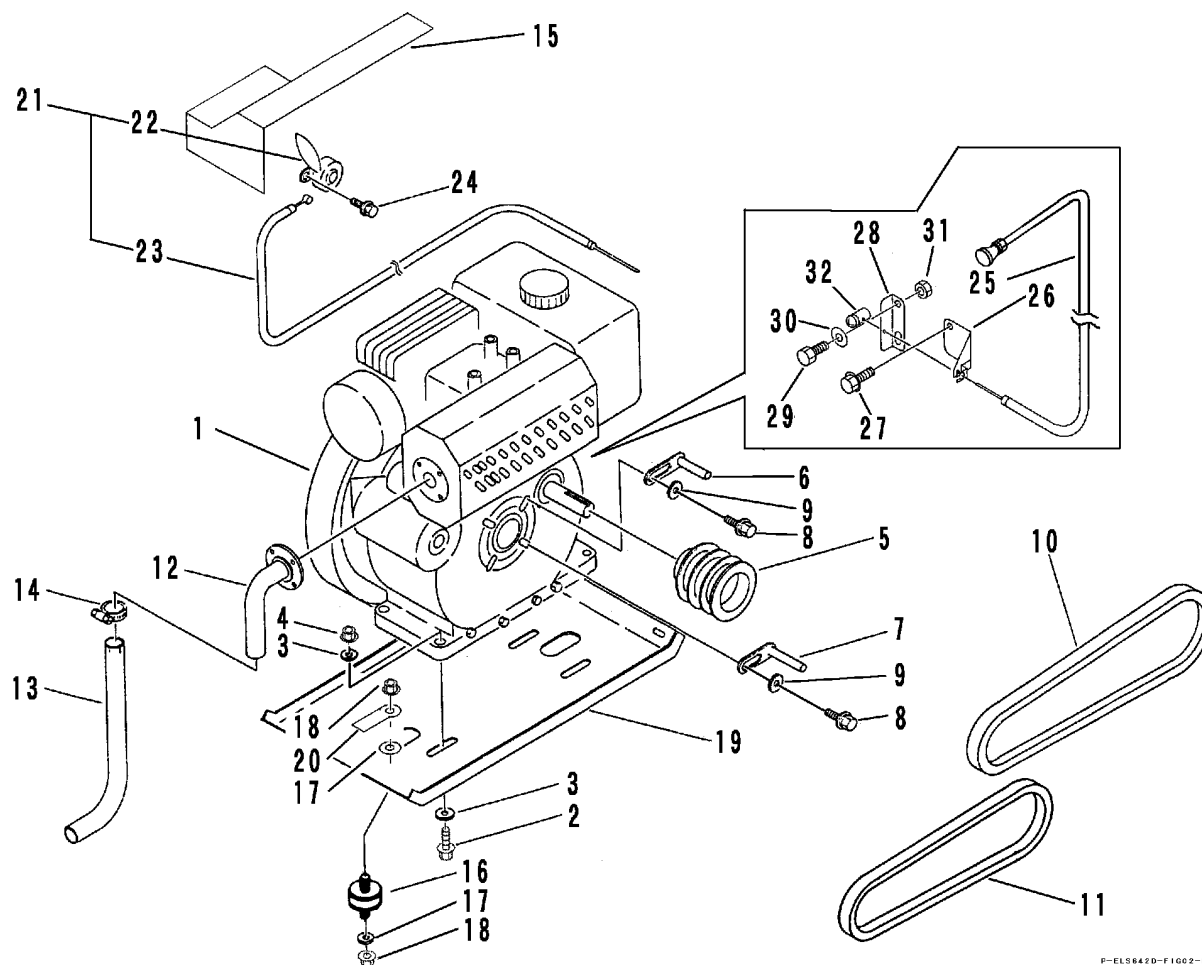
FIG 2 エンジン & エンジンコントロール (クボタ ディーゼル) ENGINE & ENGINE CONTROL
