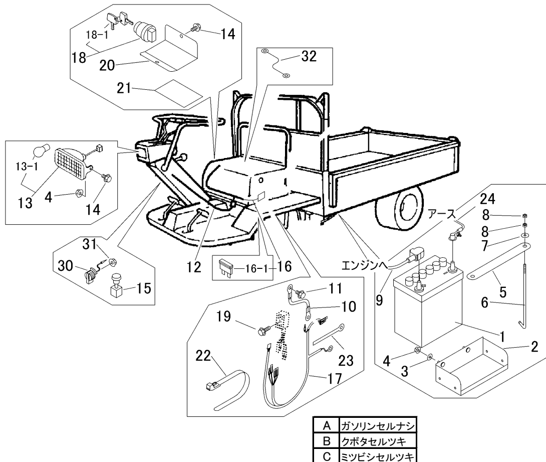
FIG 3 デンソウ (三菱シ・クボタ ガソリン) ELECTRIC EQUIPMENT
