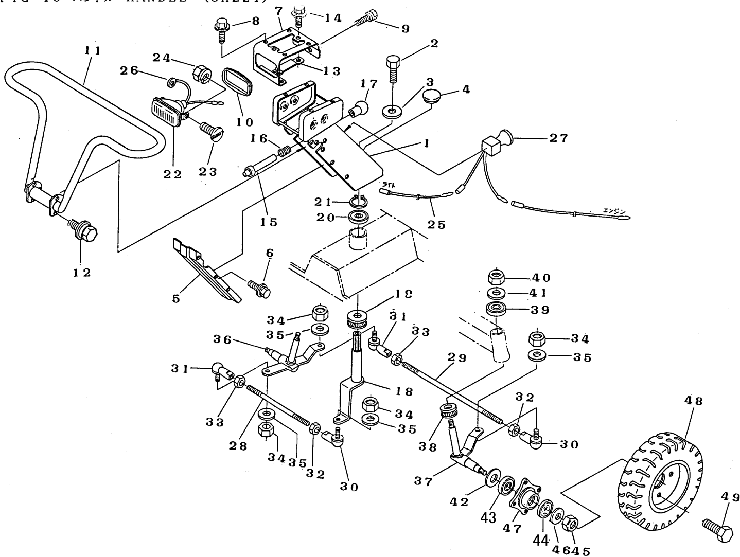
FIG 10 ハンドル HANDLE (GH221)
