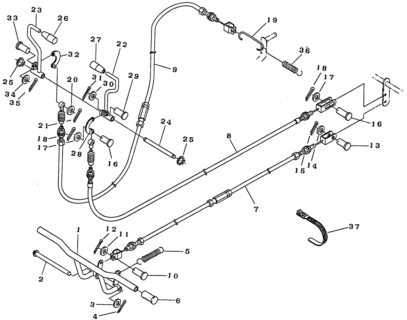
Fig 12ブレーキ
