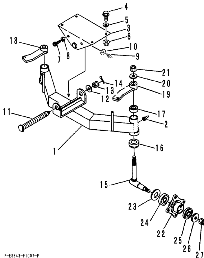
FIG 5 マエシャジク FRONT AXLE
