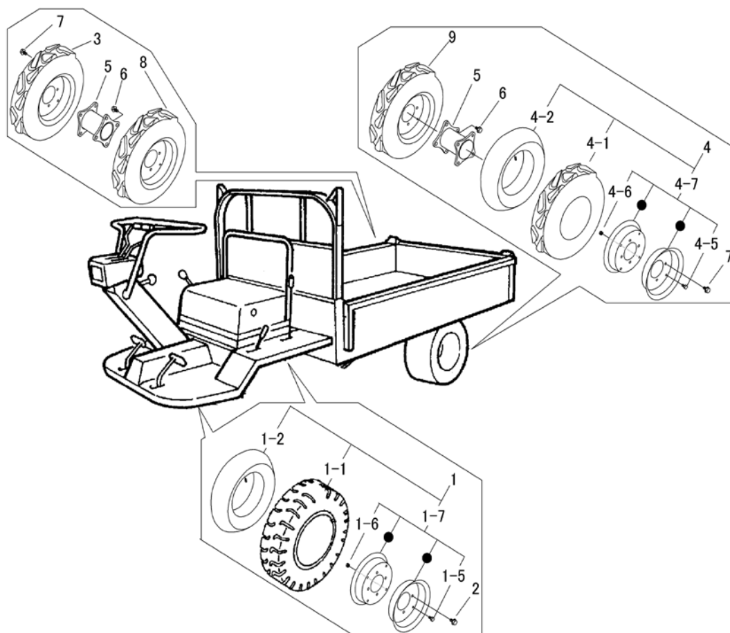
FIG 6 タイヤ TIRE
