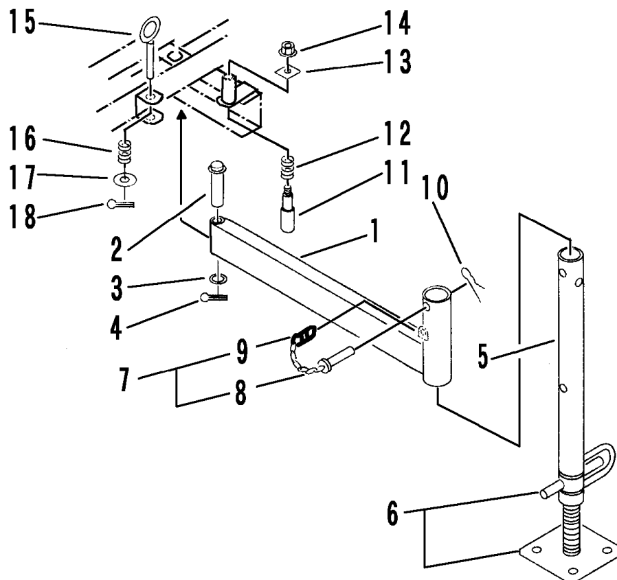
FIG 18 アウトリガー OUTRIGGER
