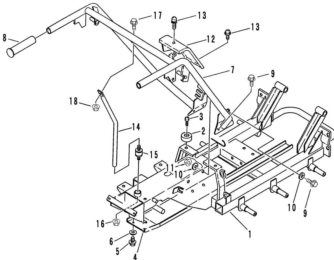
FIG 4 フレーム & ハンドル (手動ダンブ) FRAME & HANDLE (Manual hand tipping)
