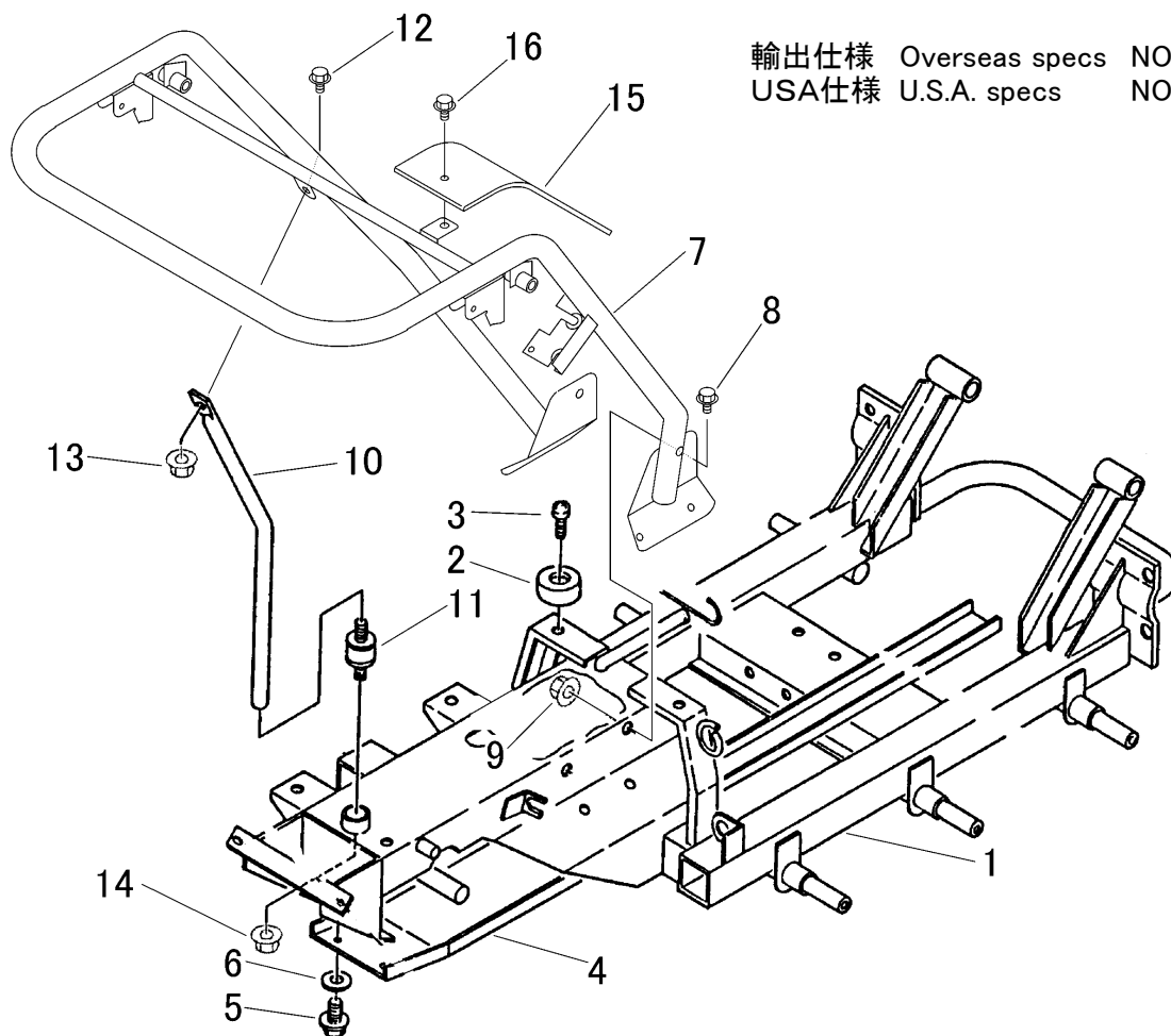
FIG 4-1 フレーム & ハンドル (手動ダンプ) FRAME & HANDLE (Manual hand tipping)
