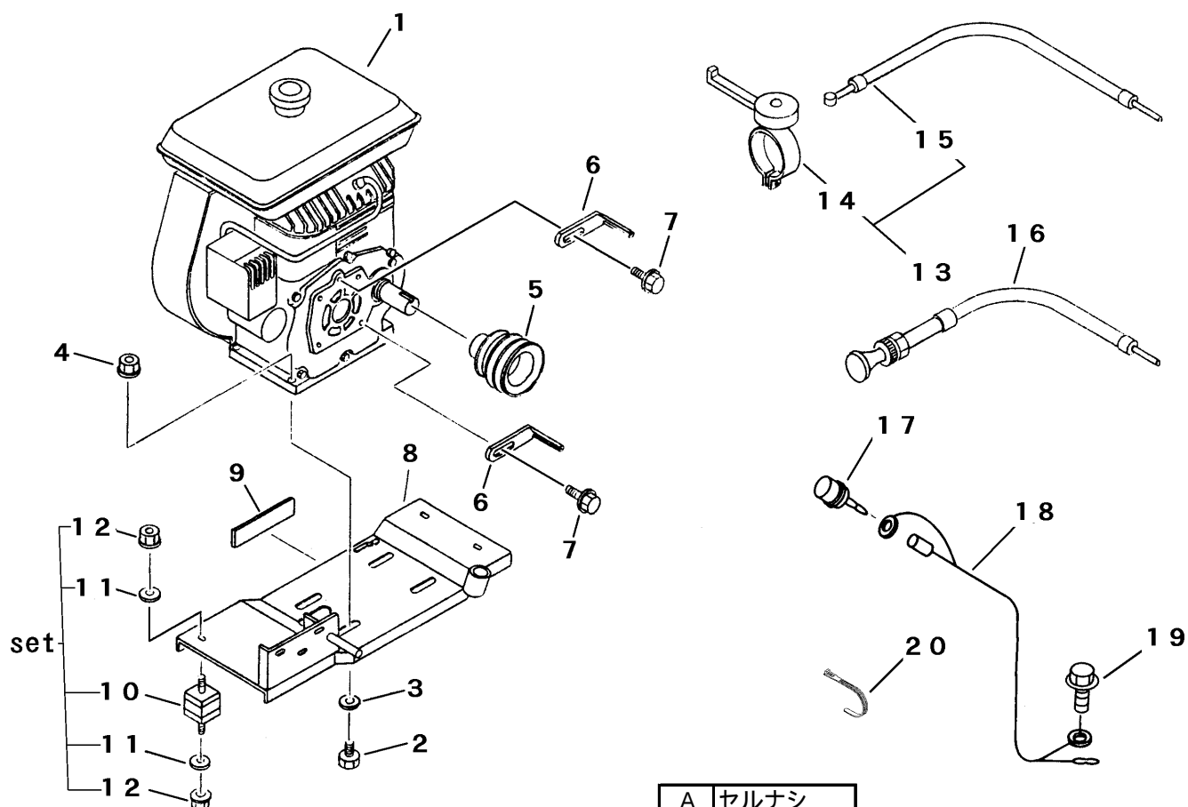
FIG 1 エンジン & エンジンコントロール ENGINE & ENGINE CONTROL
