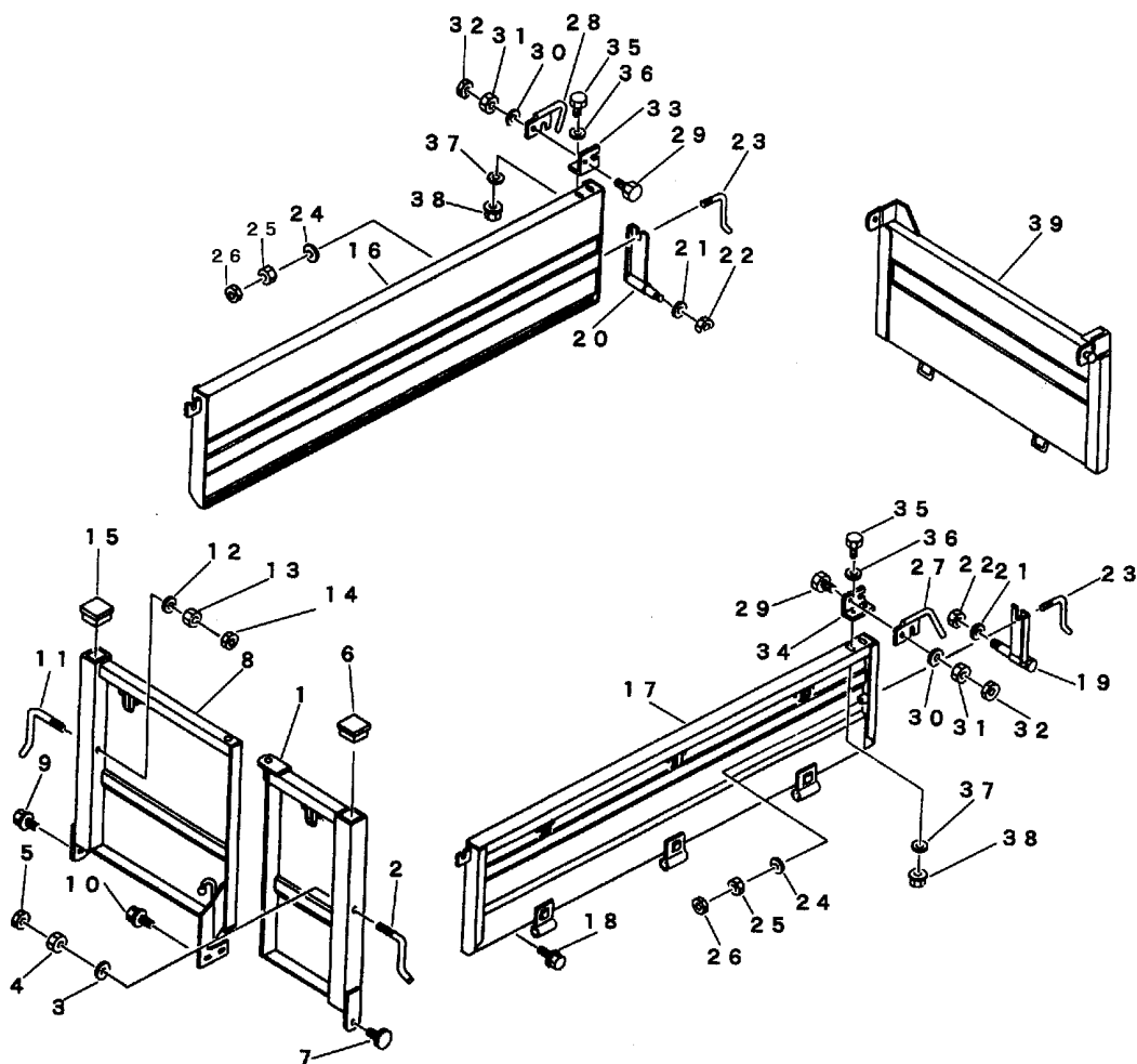
FIG 12 ドア (リフト &amp; ダンプ) GATE (LIFT &amp; DUMP)
