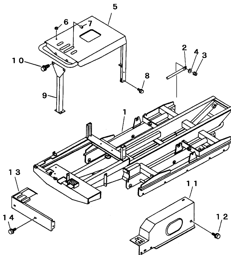
FIG 3 フレーム & エンジンカバー FRAME & COVER
