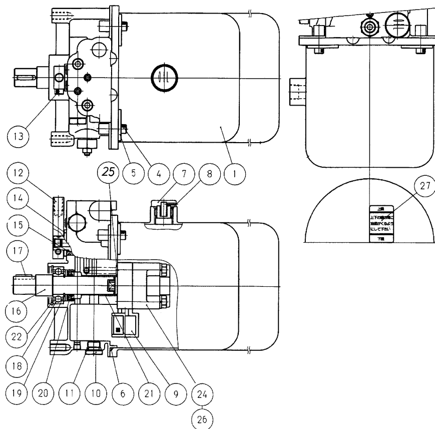
FIG 21 パッケージ (深荷箱ダンプ) HYDRAULIC PUMP NO.7740331 ~
