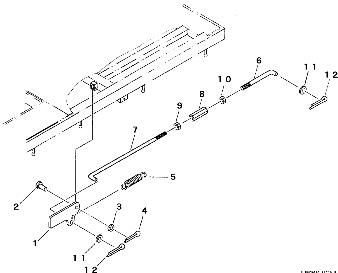
FIG 15 ドアロック LOCK
