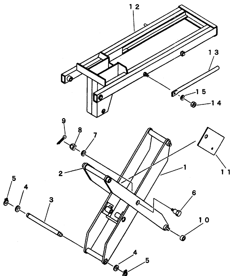
FIG 11 クロスバー (リフト &amp; ダンプ) CROSS BAR (LIFT &amp; DUMP)
