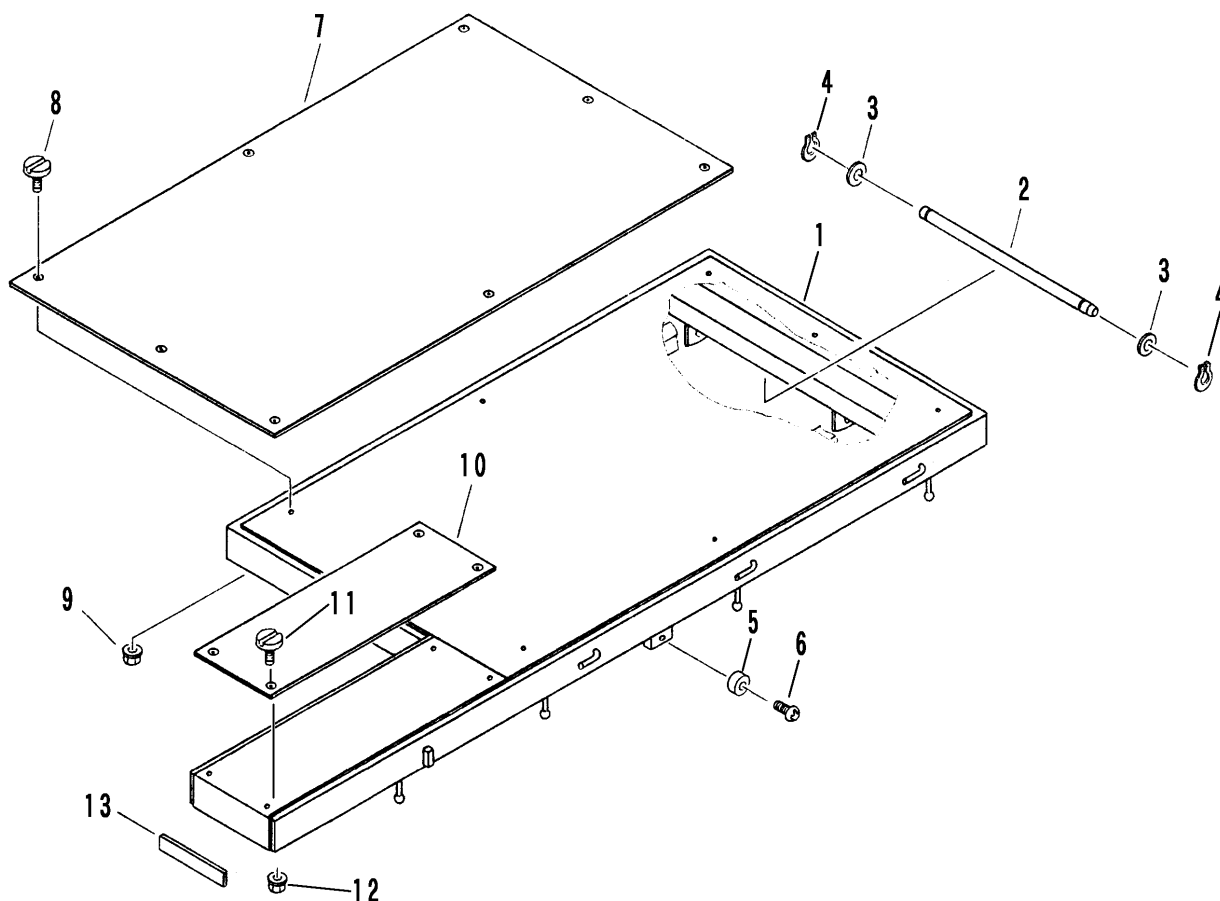
FIG 10 ニダイ (リフト &amp; ダンプ) WAGON (LIFT &amp; DUMP)
