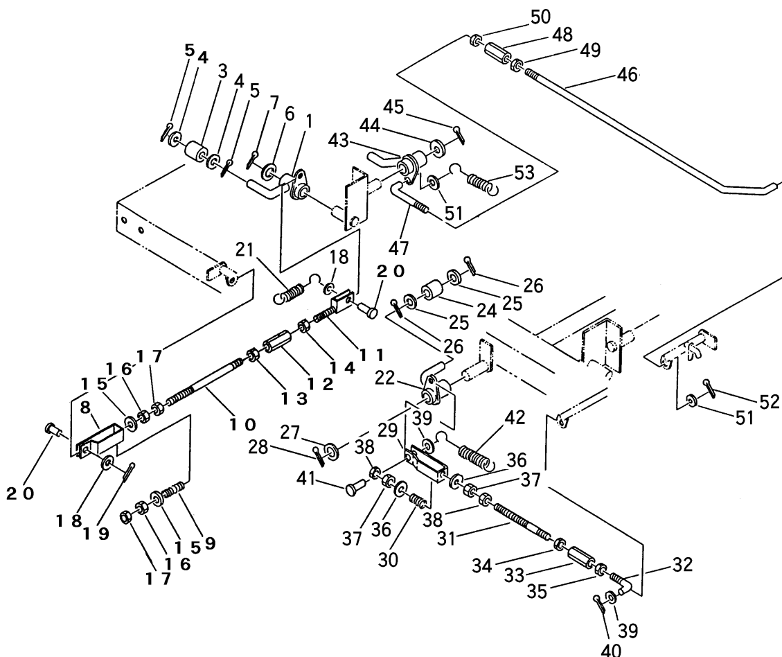
FIG 25 ドアロックソウチ GATE LOCK
