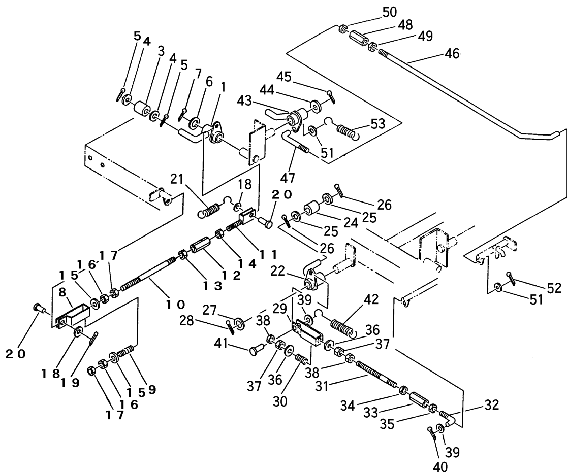
FIG 25 ドアロックソウチ GATE LOCK
