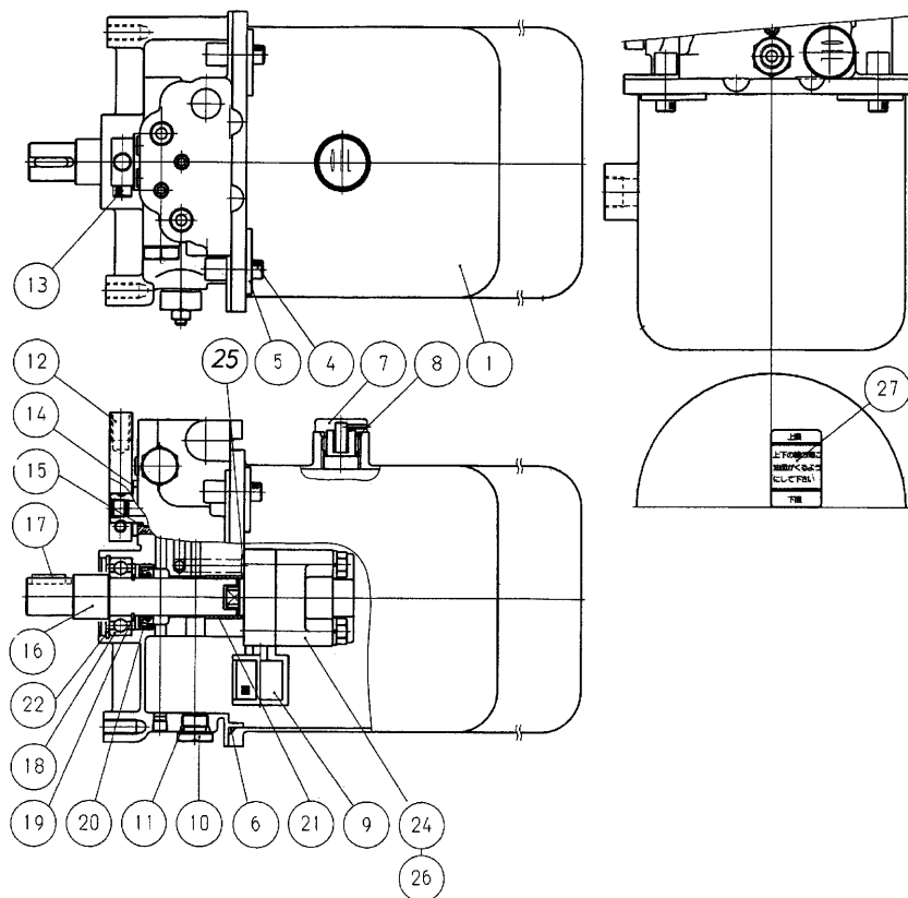
FIG 27-1 パッケージ (パワステなし) HYDRAULIC PUMP ( 補修用 ) NKPU-50-L-02 ( 樹脂製タンク )
