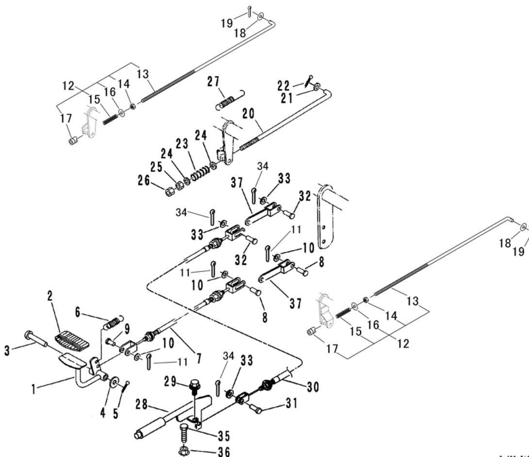
FIG 14 ブレーキ BRAKE
