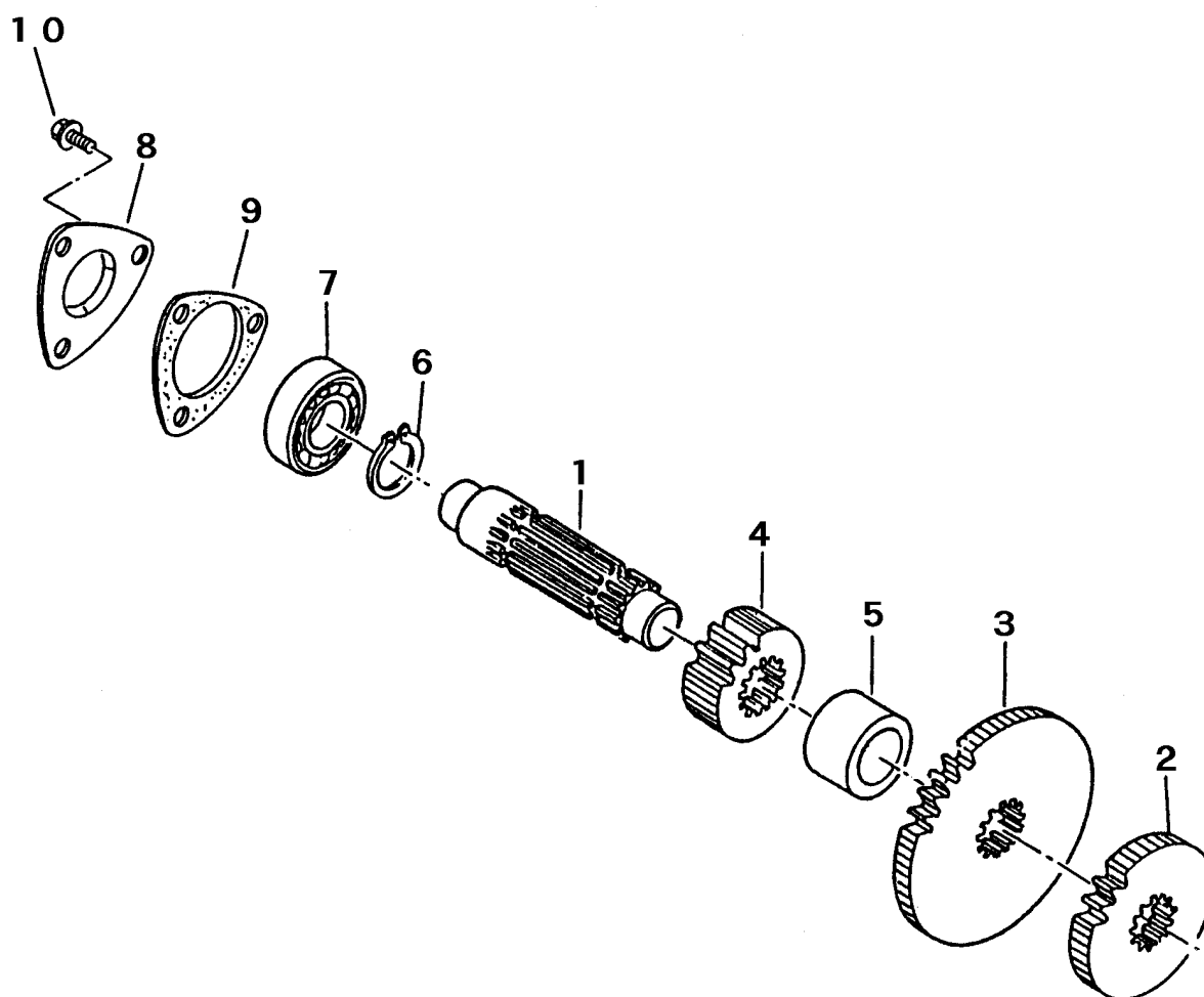
FIG 3 バックシャフト BACK SHAFT
