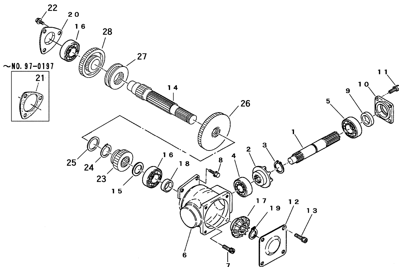
FIG 2 ニュウリョクジク DRIVE SHAFT
