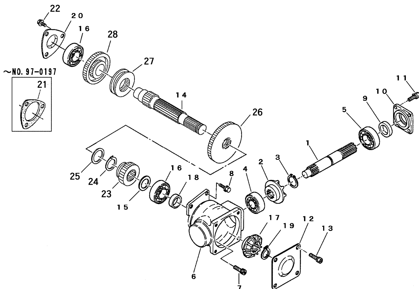
FIG 2 ニュウリョクジク DRIVE SHAFT
