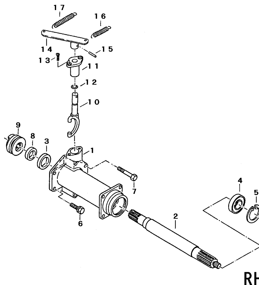
FIG 8 アクスル ライト RIGHT AXLE SHAFT
