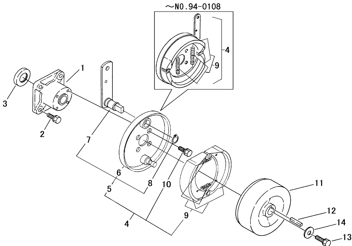
FIG 10 ブレーキ BRAKE
