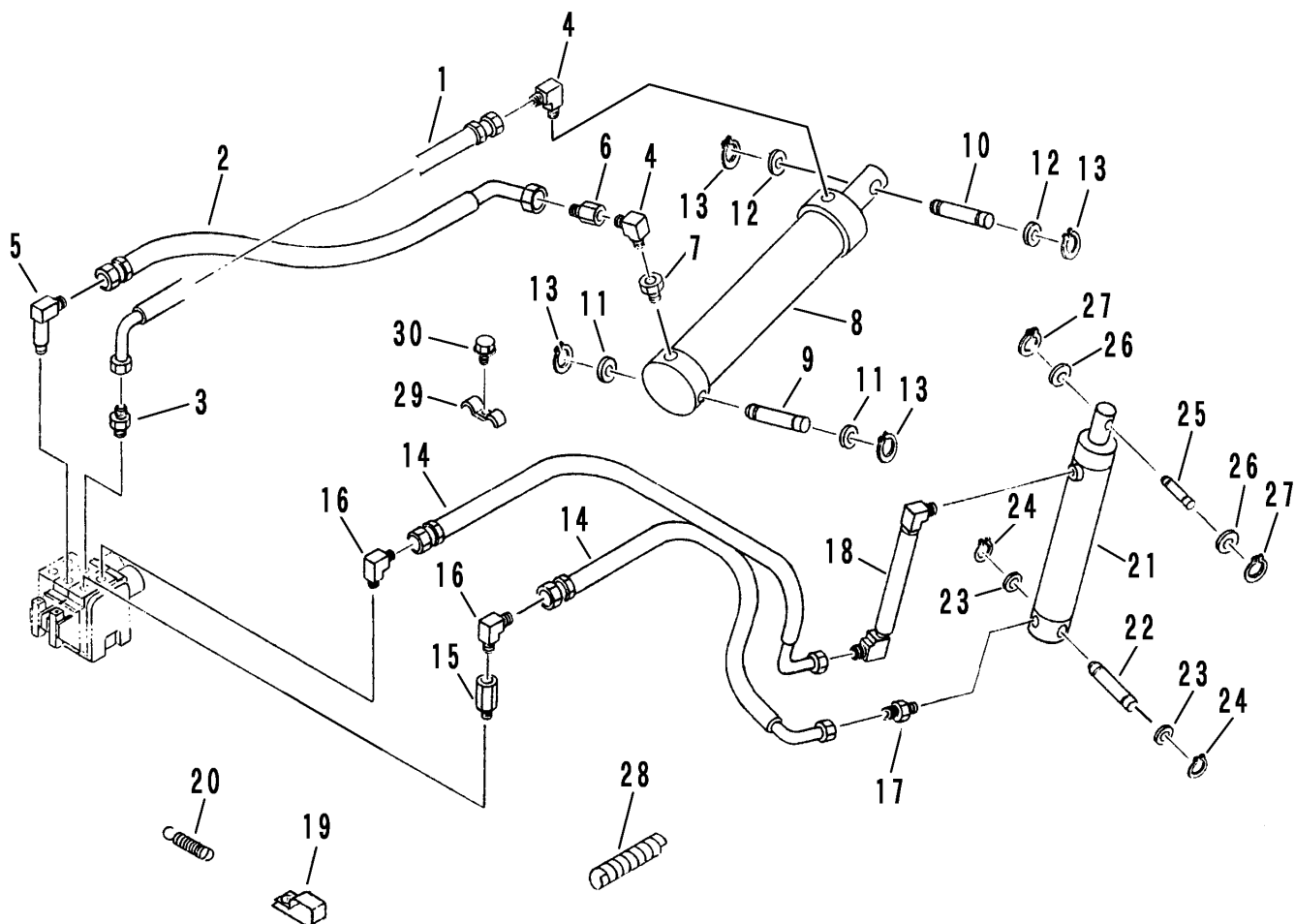
FIG 18 シリンダー CYLINDER
