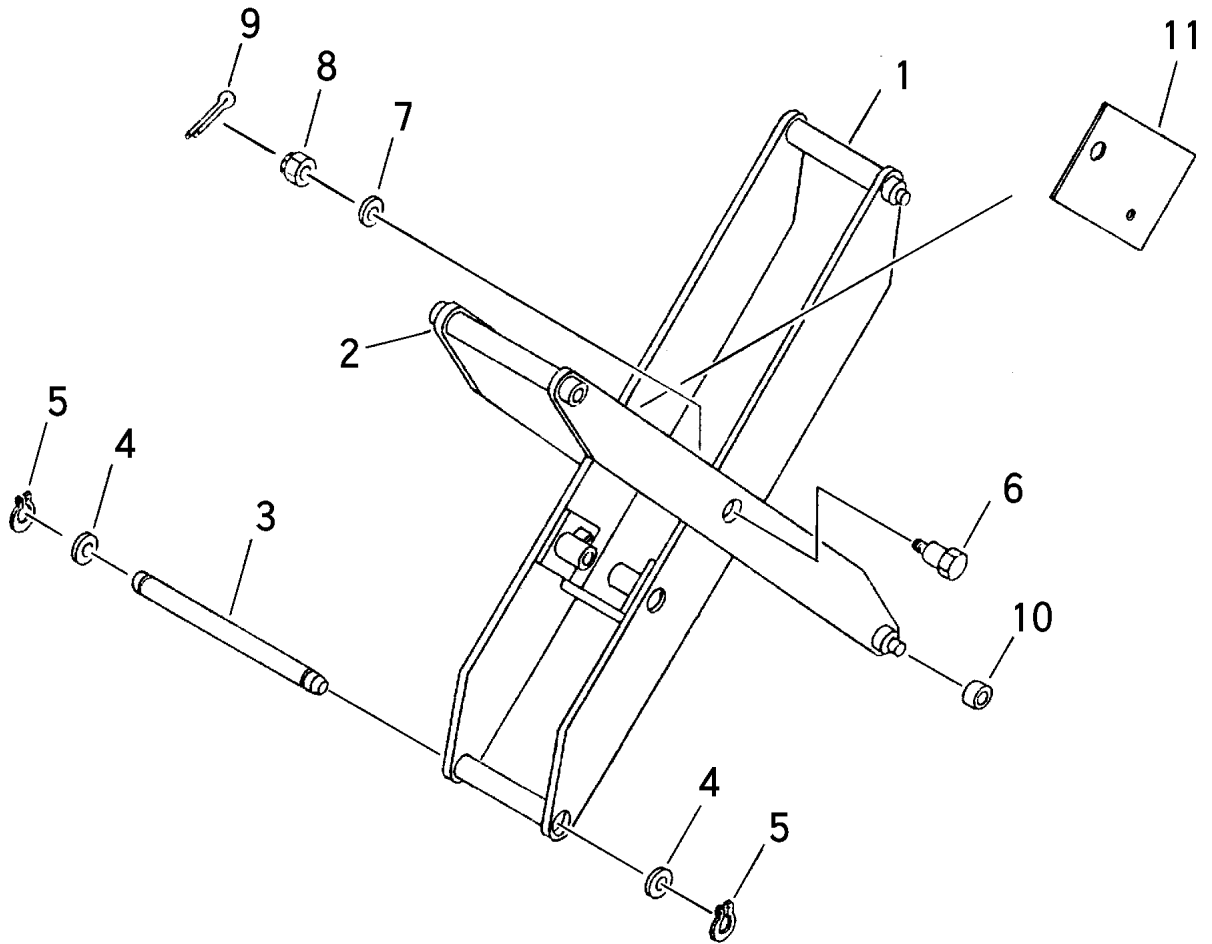
FIG 13 クロスバー CROSS BAR
