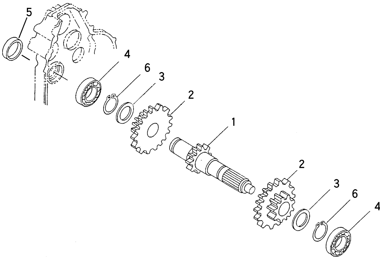
FIG 6 ブレーキジク BRAKE SHAFT
