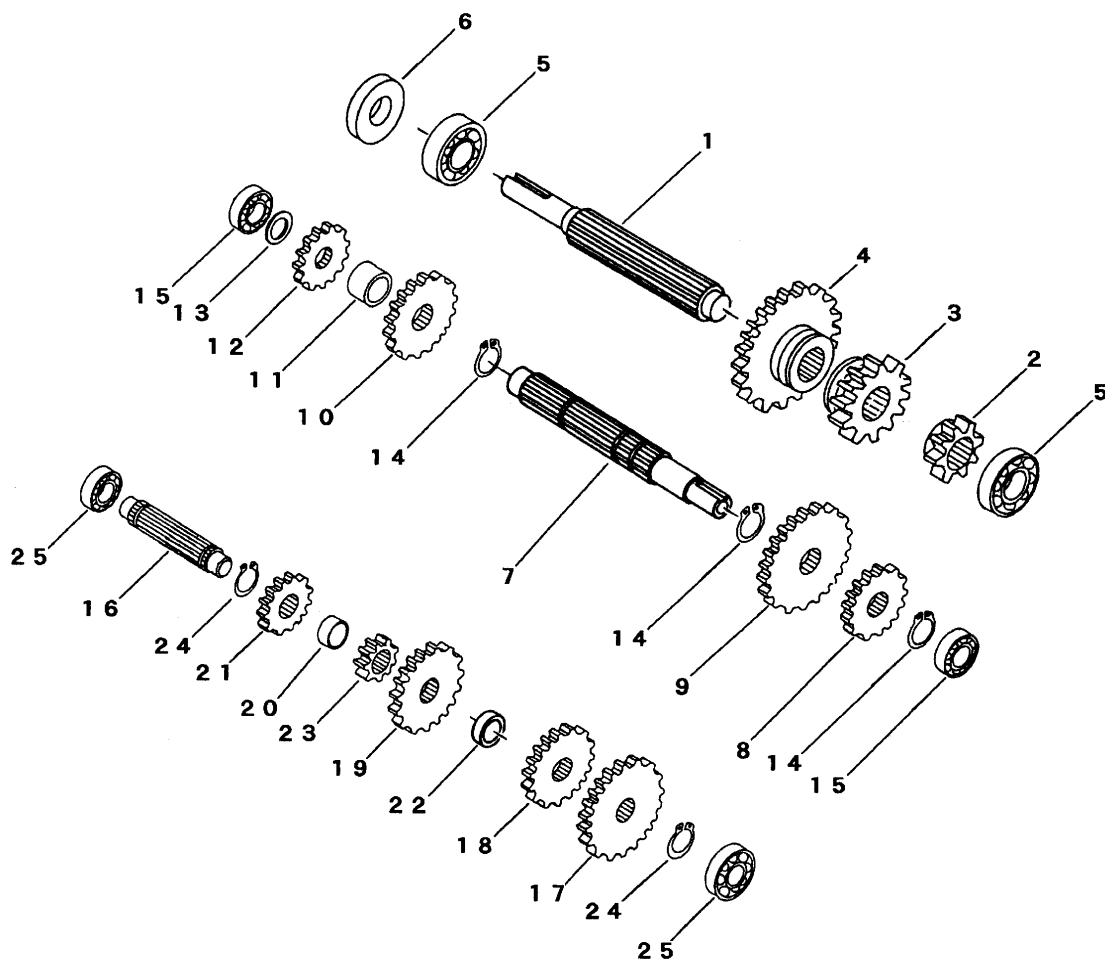
FIG 2 シャフト SHAFT
